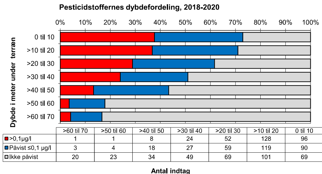
Figur 51. GRUMO. Pesticidstoffers dybdefordeling for GRUMO-indtag prøvetaget i 2020 og for perioden 2018-2020. Indtagene er opdelt i tre koncentrationsintervaller: >0,1 µg/l, påvist ≤0,1 µg/l, samt ikke påvist (under detektionsgrænsen, typisk <0,01 µg/l). Dybden angiver afstanden fra terræn til overkanten af indtaget.
