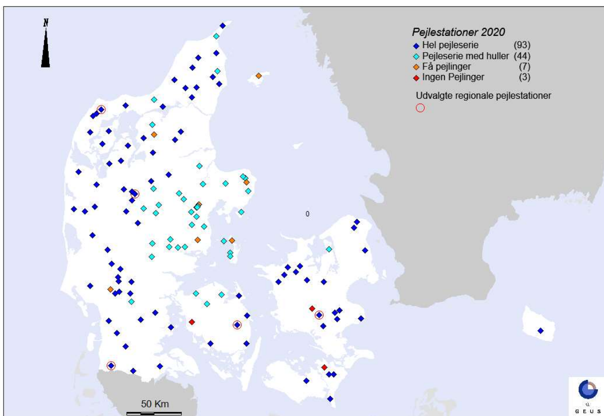
Figur 63. Beliggenhed af de 147 indtag i pejlestationsnettet, fordelt på 138 borer, som indgik i Det nationale Pejleprogram i 2020, herunder de 5 udvalgte regionale pejlestationer med lange tidsserier.
