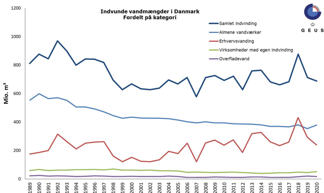
Figur 1. Vandindvinding i Danmark i perioden 1989-2020 opdelt på almene vandværker, erhvervsvandning, industri og overfladevand. Med en fed, mørkeblå linje er den samlede indberettede indvinding vist. Bemærk, hvorledes den varierer med erhvervsvandningen, hvoraf markvandingen udgør hovedparten.
