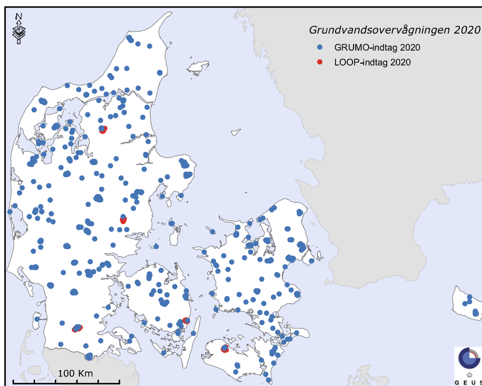
Figur 66. GRUMO. Indtag anvendt i grundvandsovervågningen i 2020 fordelt på grundvandsovervågning (806 GRUMO-indtag) og landovervågning (91 LOOP-indtag).
