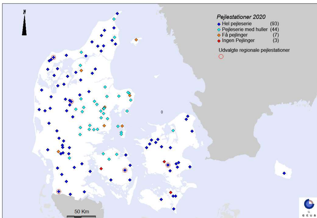
Figur 17. Geografisk fordeling af de 147 stationer, der indgik i Det nationale Pejlenet 2020, inklusiv 5 udvalgte regionalt udvalgte pejlestationer med lange tidsserier.
