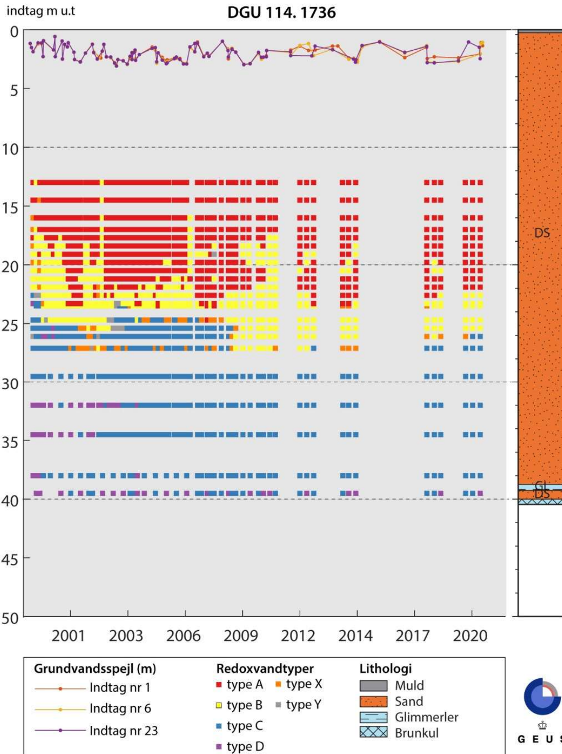
Figur 35. Grindsted i Midtjylland, DGU nr. 114.1736 med redoxvandtyper for perioden 1999-2020. Grundvandsspejlet er beliggende i ca. 2 m u.t. Det geologiske profil er vist længst til højre på figuren.
