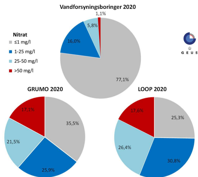
Figur 2. GRUMO, LOOP og Vandforsyning. Fordelingen af det gennemsnitlige nitratindehold 2020 i 806 GRUMO-, 90 LOOP-indtag og 1.608 vandforsyningsboringer.
