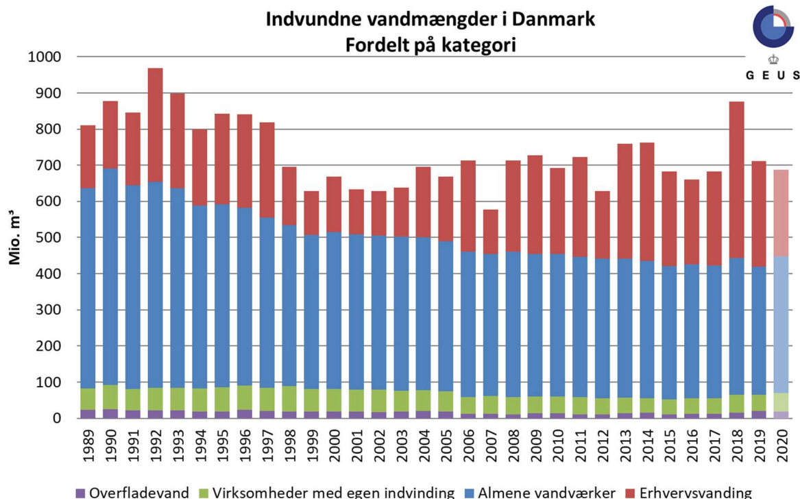
Figur 15. Vandindvinding i Danmark i perioden 1989-2020 opdelt på almene vandværker, erhvervsvanding, industri og overfladevand. Data fra 2020 er justeret med skøn over manglende rapportering og er vist med nedtonede farver.
