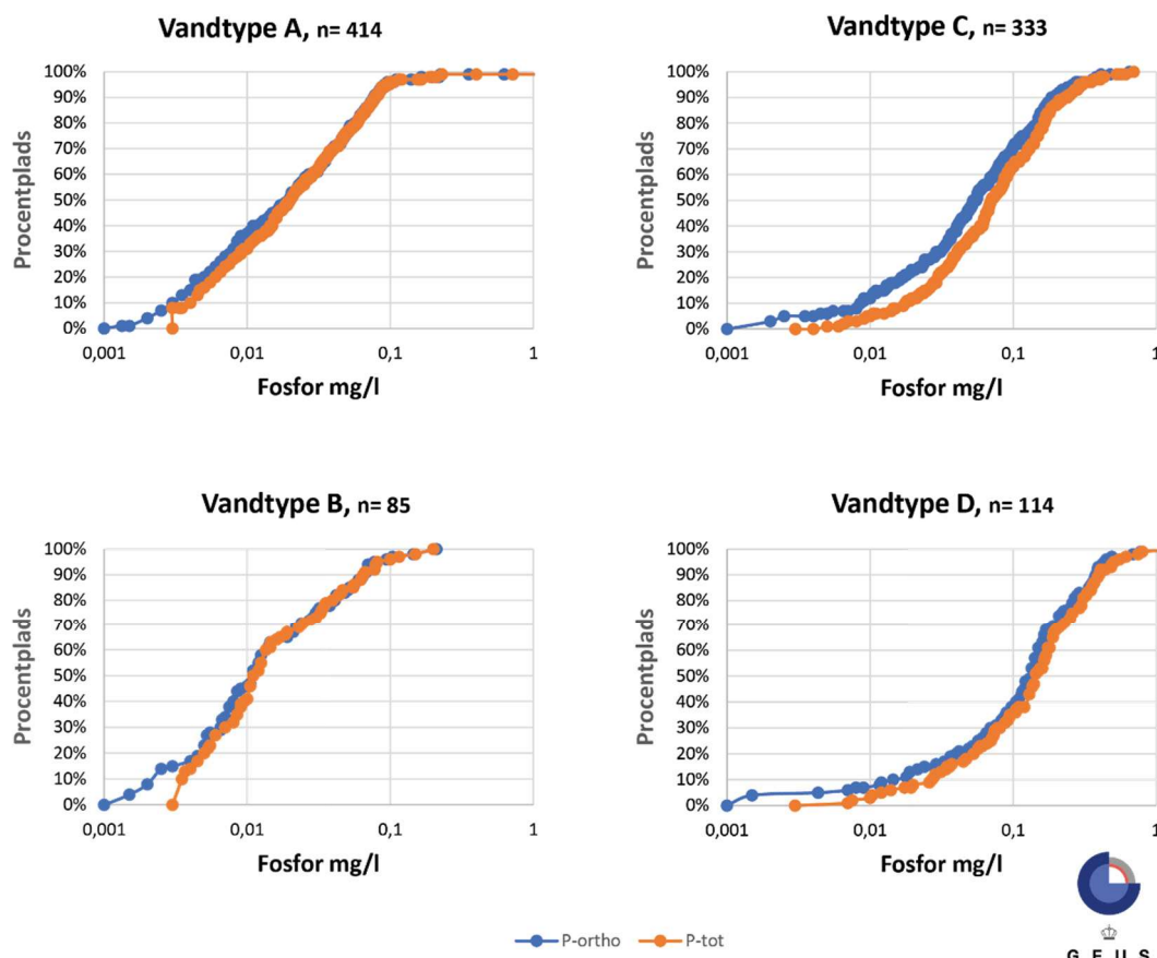
Figur 43. GRUMO. Koncentrationsfordelingen for det gennemsnitlige fosforindhold i GRUMO-indtag for re-doxvandtype A-D for P_{tot} og P_{ortho} for perioden 2019-2020. Antal indtag (n) for hver redoxvandtype. Bemærk, der er anvendt en logaritmisk skala.
