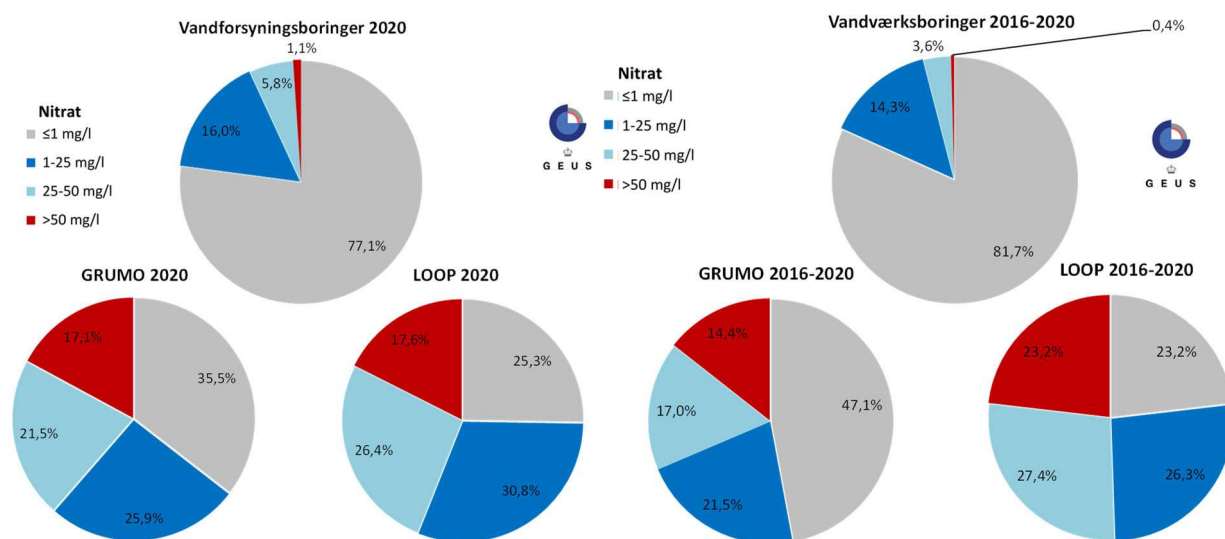
Figur 22. GRUMO, LOOP & Vandforsyning. Fordelingen af det gennemsnitlige nitratinhold pr. indtag i 2020 for 806 GRUMO-indtag, 91 LOOP-indtag og 1.607 vandforsyningsboringer og i perioden 2016-2020 for 1.277 GRUMO-indtag, 95 LOOP-indtag og 6.111 vandforsyningsboringer.
