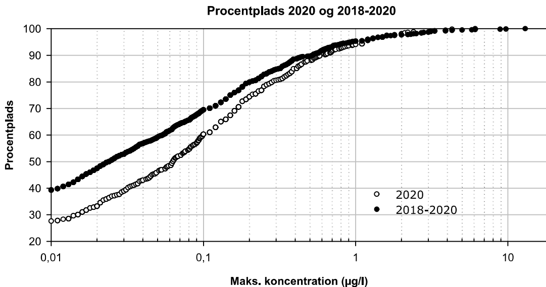
Figur 50. GRUMO. Procentpladsfordeling for højest målte pesticidkoncentration opgjort for GRUMO-indtag prøvetaget i 2020 og i perioden 2018-2020. Det fremgår, at i 2020 blev der ikke påvist pesticider i 27,6 % af de undersøgte indtag, og i perioden 2018-2020 i 39,0 % af de undersøgte indtag.
