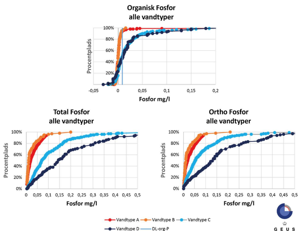
Figur 44. GRUMO. Koncentrationsfordelingen for det gennemsnitlige fosforindhold i GRUMO-indtag for redoxvandtype A-D for P_{\text{tot}} og P_{\text{ortho}} og P_{\text{org}} for perioden 2019-2020. Antal indtag for hver redoxvandtype fremgår af Figur 43.
