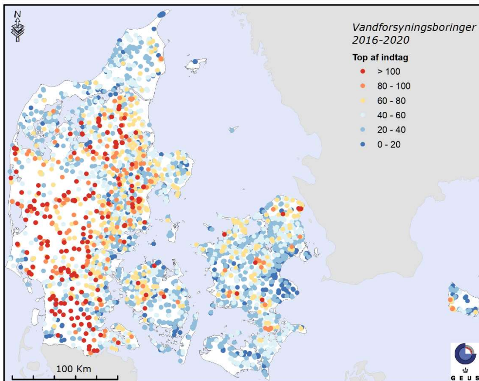
Figur 71. Vandforsyning. Dybde til toppen (m u.t.) af indtag for vandforsyningsboringer i perioden 2016-2020 (5.810 indtag) medkendt dybde til indtag. Data i den øverste figur er sorteret efter stigende dybde, så de korte boringer er afbildet øverst. Data i den nederste figur er sorteret efter aftagende dybde, så de dybeste boringer er afbildet øverst.
