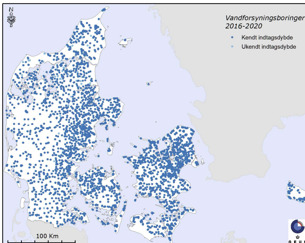
Figur 70. Vandforsyning. Den geografiske fordeling af 5.810 aktive indtag fra vandforsyningsboringer med kendt dybde til top af indtag, samt de 397 indtag med ukendt dybde til top af indtag, i perioden 2016-2020. Indtag med ukendt dybde er udtegnet nederst.
