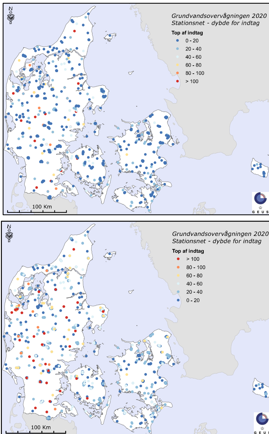
Figur 67. GRUMO. Dybde til toppen (m u.t.) af 1.298 programlagte indtag med kendt dybde i stationsnettet i grundvandsovervågningen i Danmark i 2017-2021. Data i den øverste figur er sorteret efter stigende dybde, således de mest terrænnære indtag er afbildet øverst. Data i den nederste figur er sorteret efter aftagende dybde, således de dybeste indtag er øverst på denne figur.
