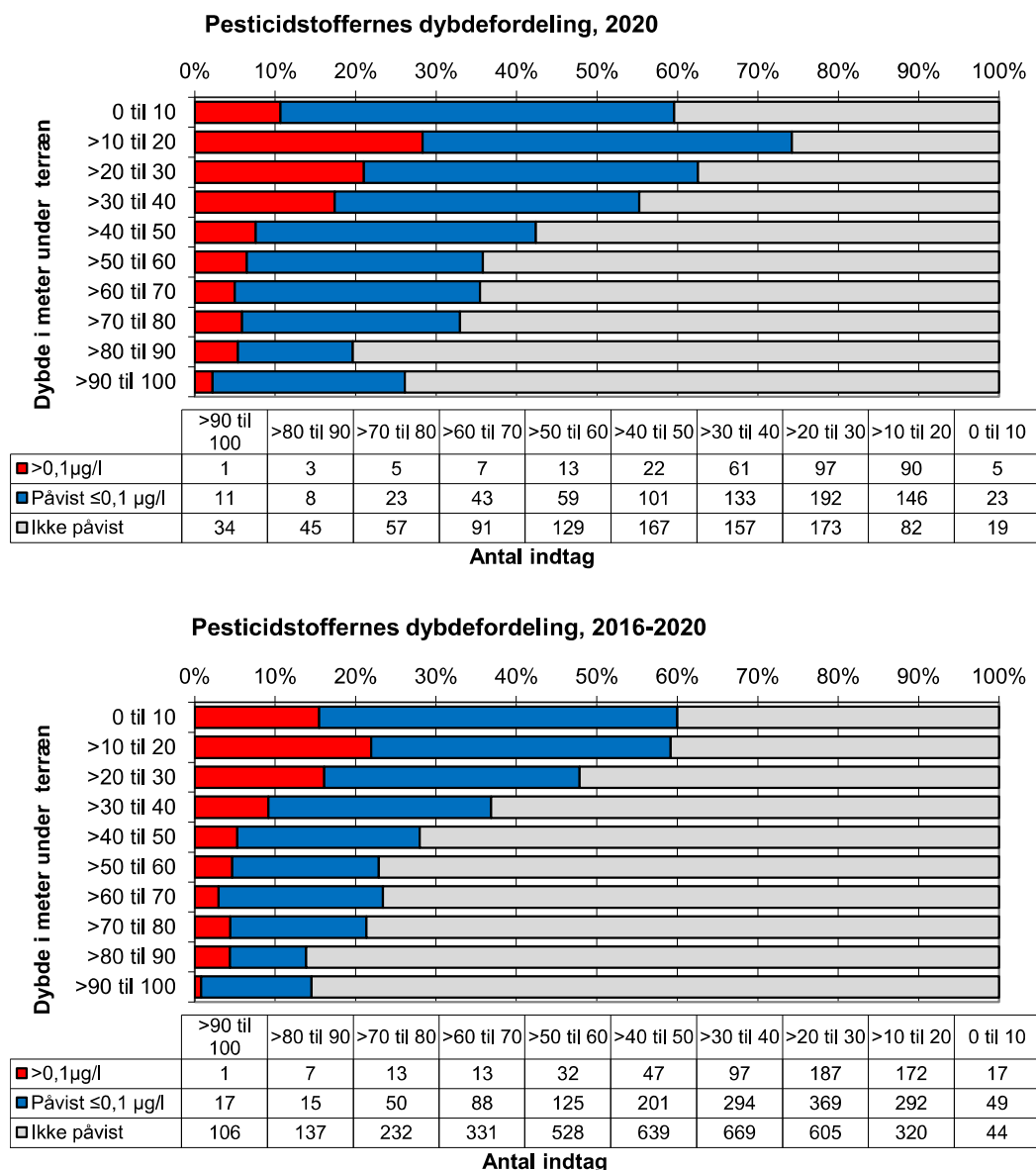
Figur 57. Vandforsyning. Pesticidstoffers dybdefordeling for indtag prøvetaget i 2020 og for perioden 2016-2020. Indtagene er opdelt i tre koncentrationsintervaller: >0,1 µg/l, påvist ≤0,1 µg/l, samt ikke påvist (under detektionsgrænsen, typisk <0,01 µg/l). Dybden angiver afstanden fra terræn til overkanten af indtaget.
