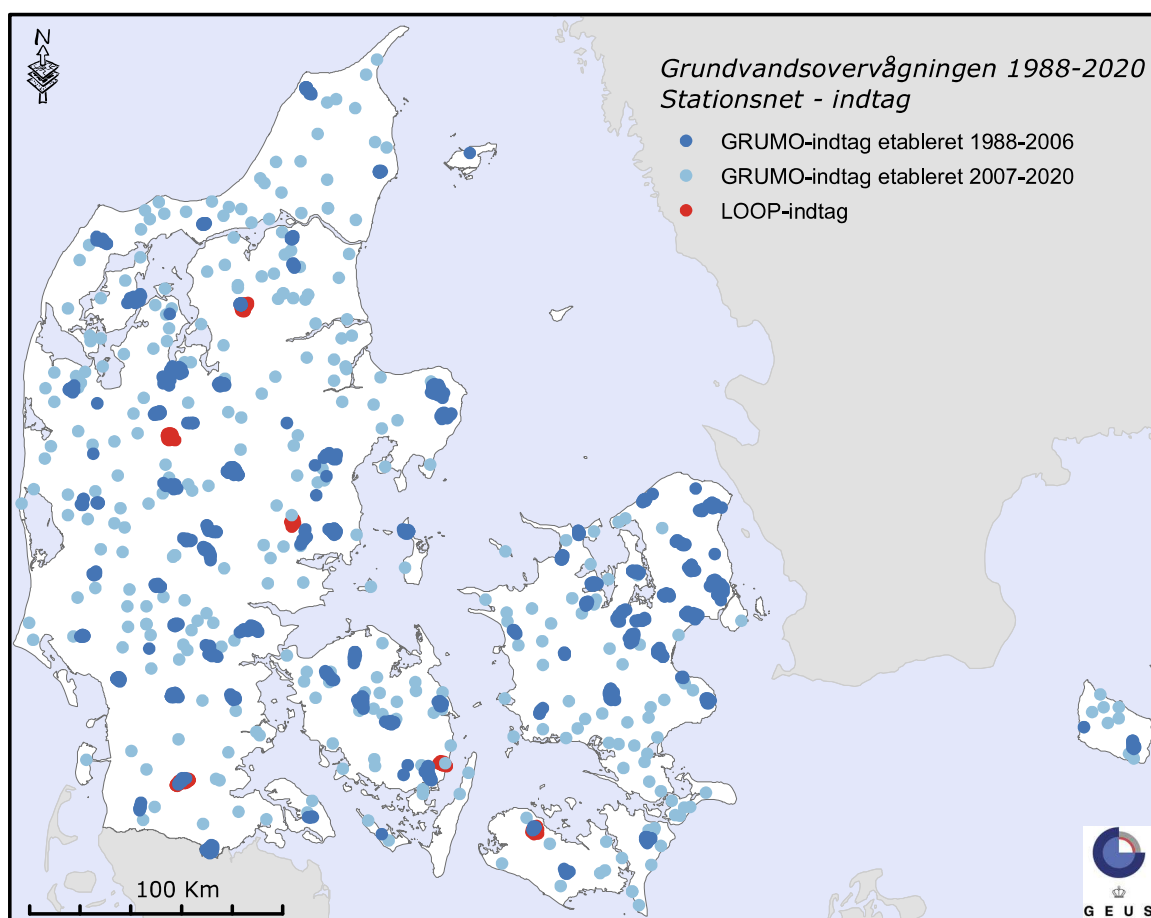
Figur 64. GRUMO. Det samlede stationsnet i grundvandsovervågningen i Danmark i perioden 1988-2020. Kortet viser indtag i de oprindelige 73 grundvandsovervågningsområder (GRUMO-indtag 1988-2006) og indtag i overvågningsboringer i det distribuerede stationsnet (GRUMO-indtag 2007-2020). Desuden ses LOOP-indtagene i de seks landovervågningsoplande, hvoraf det ene i Midtjylland ved Herning er lukket.
