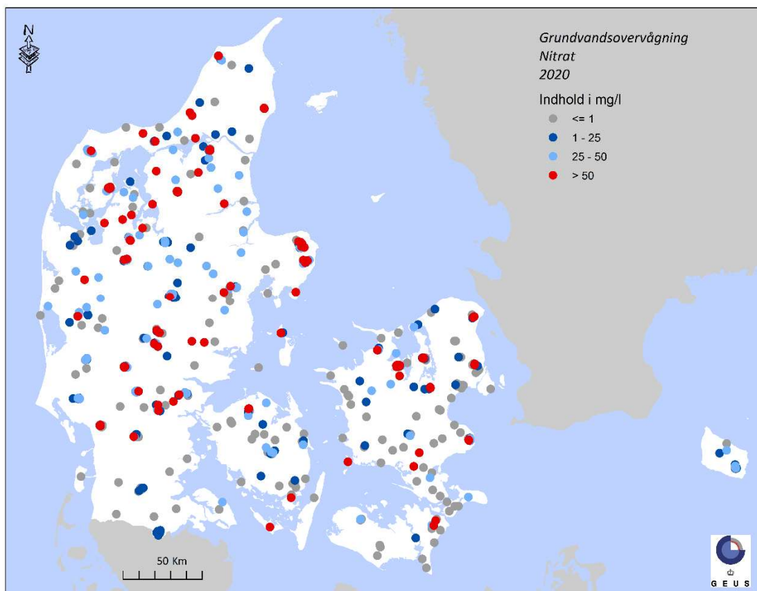
Figur 3. GRUMO. Nitratindeholdet i grundvand i 2020 i 805 GRUMO-indtag. Nitratindeholdet er opdelt på fire koncentrationsklasser. De højeste koncentrationer er afbildet øverst.
