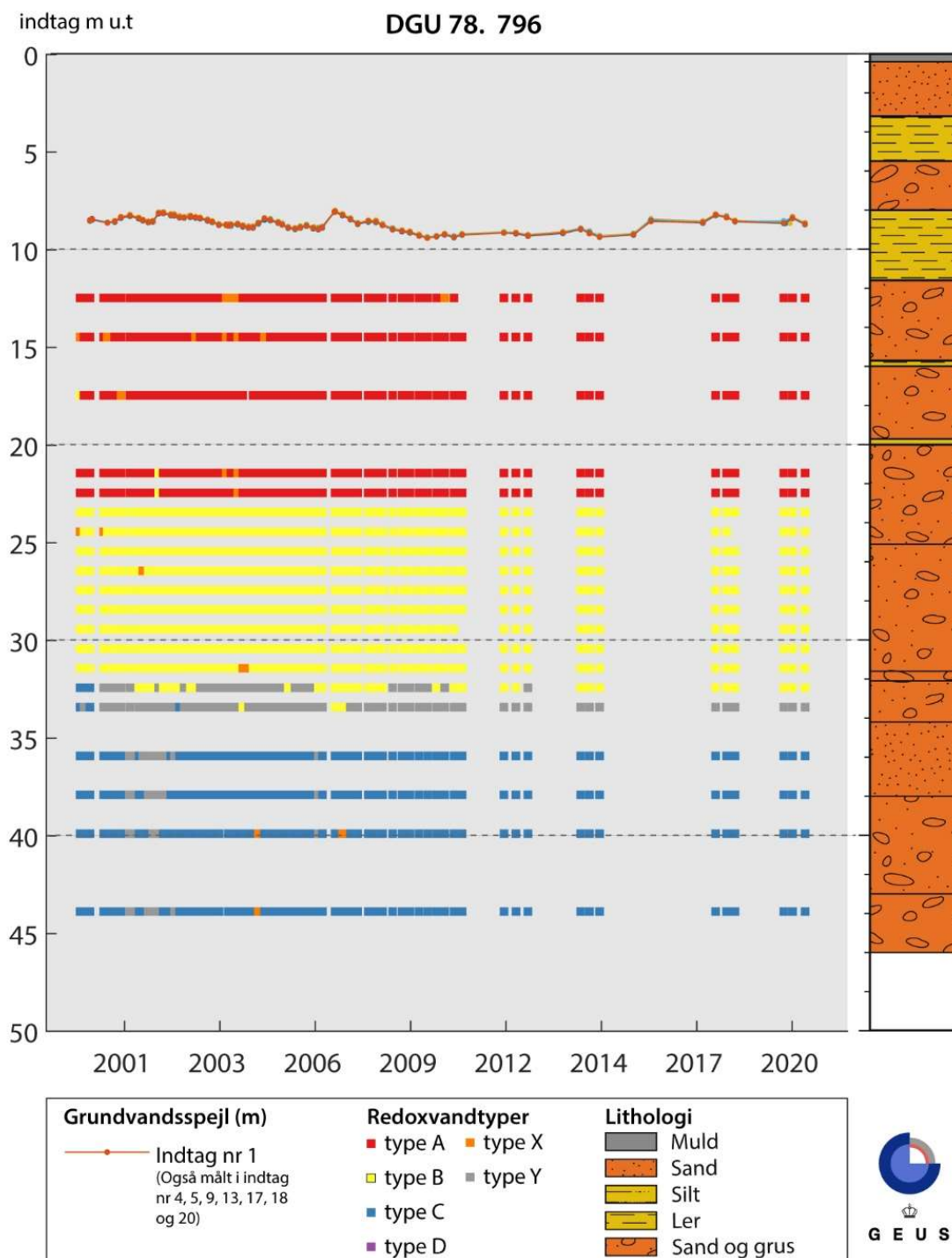
Figur 34. Kasted nordvest for Århus, DGU nr. 78.796, med redoxvandtyper for perioden 1999-2020. Grundvandsspejl i ca. 9 m u.t. Det geologiske profil er vist længst til højre på figuren.
