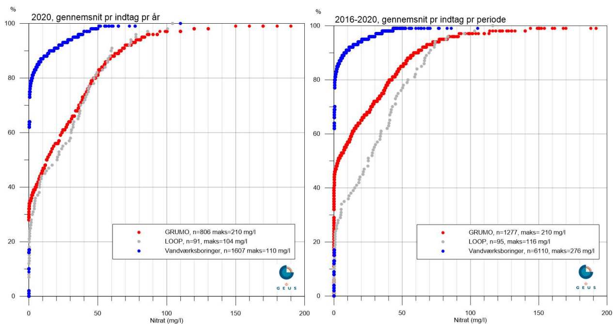
Figur 23. GRUMO, LOOP & Vandforsyning. Fordelingen af det gennemsnitlige nitratinhold i grundvandet i 2020 (venstre del af figuren) og i perioden 2016-2020 (højre del af figuren) i alle indtag fra GRUMO- og LOOP-indtag og vandforsyningsboringer med koncentrationer under 200 mg/l. Antallet af indtag og maks. koncentration af nitrat i hver gruppe fremgår af signaturforklaringen.
